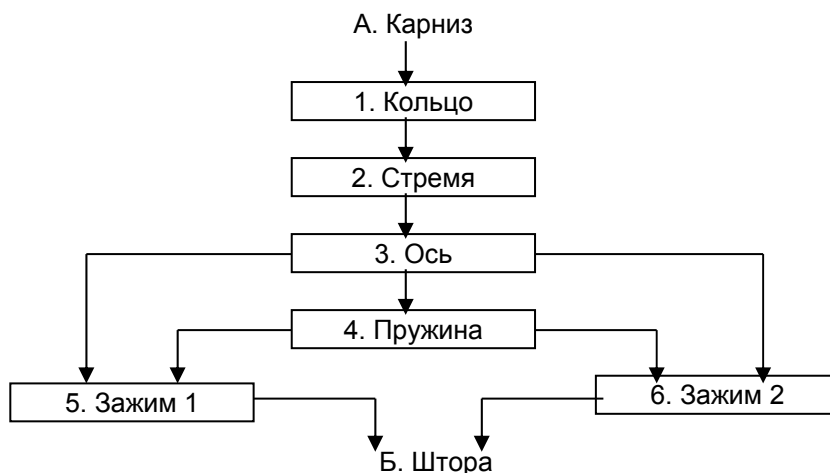
Рис. 6.23. Потоковая модель прищепки шторной
