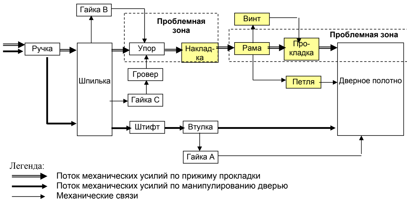
Рис. 6.14. Поточковой модели запора дверей кожуха
