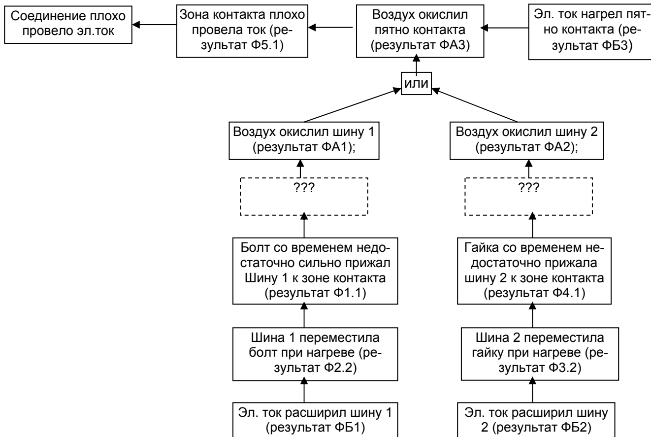
Рис. 6.21. Процесс построения ПСМ (пример, продолжение)
