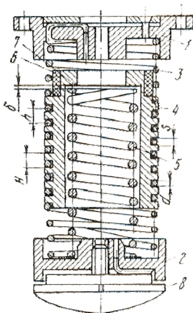
Рис. 7.9. Амортизатор
