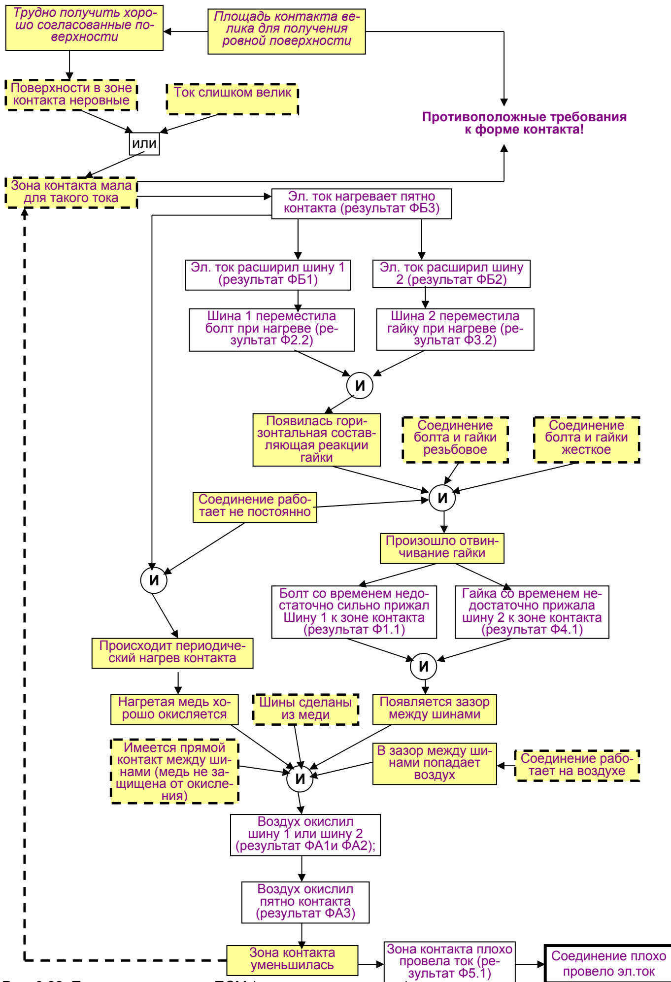
Рис. 6.22. Процесс построения ПСМ (пример, продолжение)
