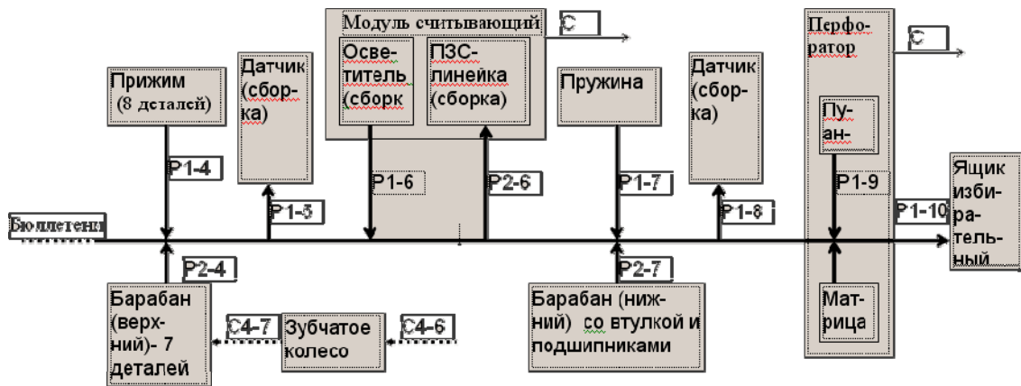
Рис. 6.13. Фрагмент укрупненной ПМВ сканера избирательных бюллетеней
