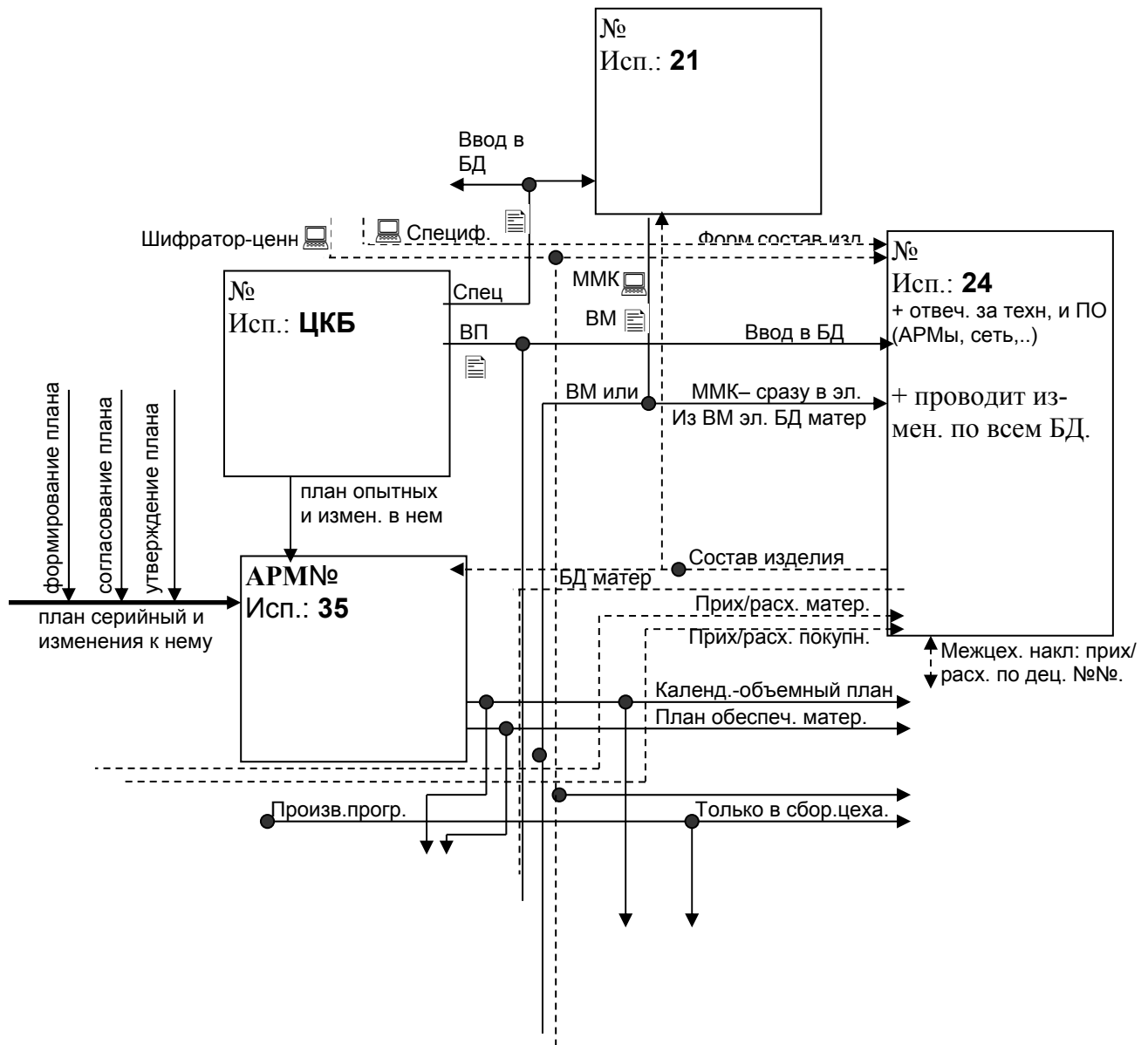
Рис. 6.15. Фрагмент ПМВ системы учета материально-технического снабжения
