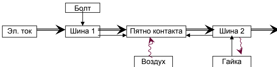
Рис. 6.17. Потокую модель болтового соединения шин
