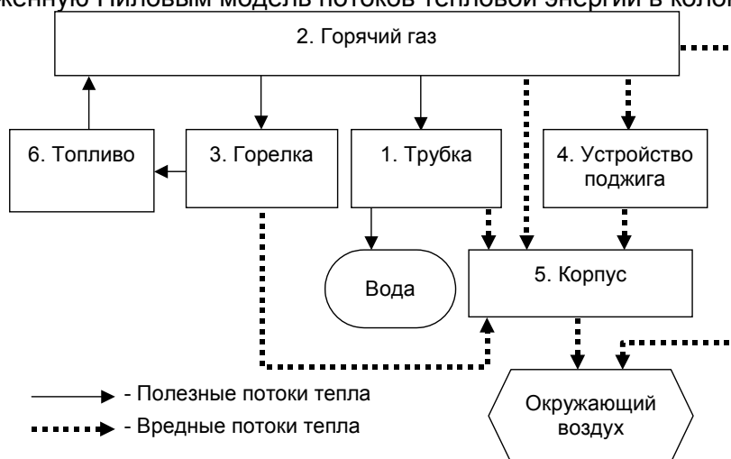
Рис. 6.8. Модель потоков тепловой энергии в теплообменнике по А.Нилову.
